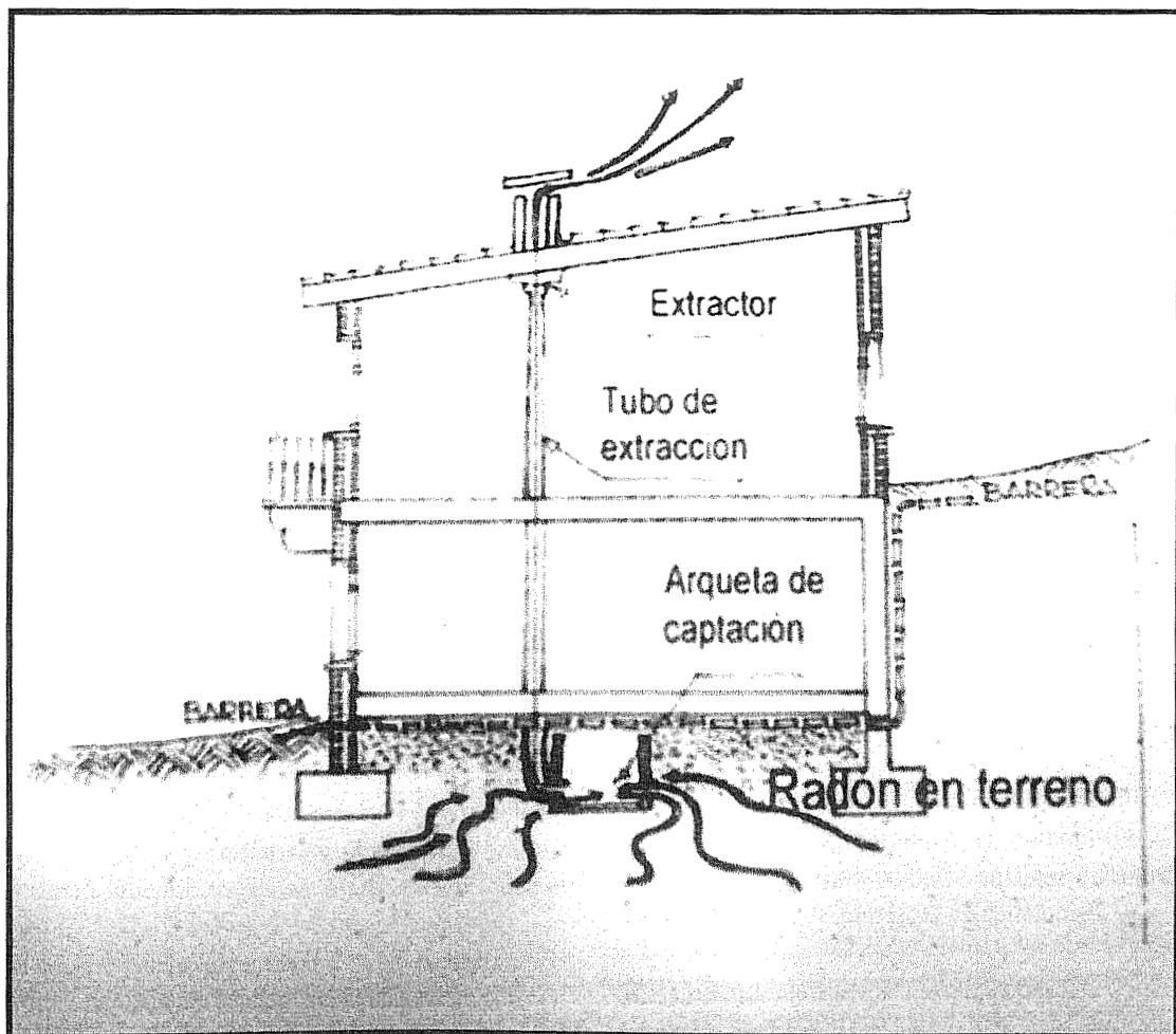
Figura nº3. Barrera bajo solera más sistema de extracción (1.S.2.1)
