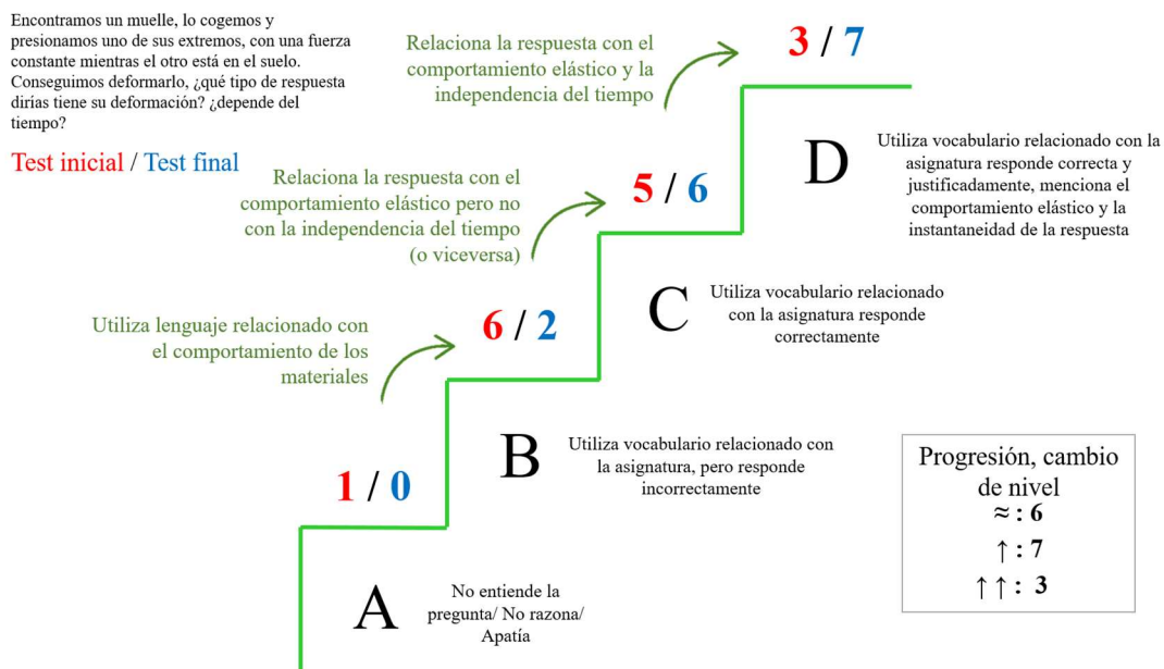
Figura 3. Escaleras de progresión de los modelos mentales de los alumnos (pregunta 1)
