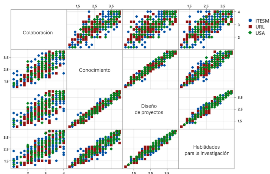
Figura 2. Gráfica de matriz entre dimensiones.
