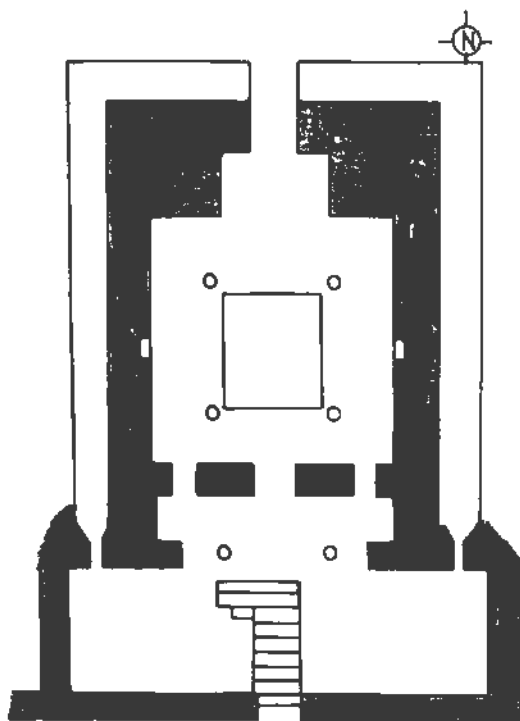
ILUSTRACION 1. Planta de la pseudodiptera de Sta. Eulalia de Bóveda (Lugo) (segun Rodriguez Colmenero, redibujado).
