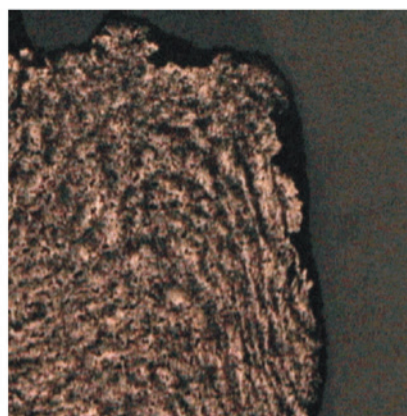
Metalografía del borde x 50.
