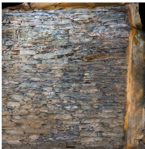
Figura 8. Detalle de la fábrica de mampuestos en el paramento norte del final del tramo intermedio del corredor.
