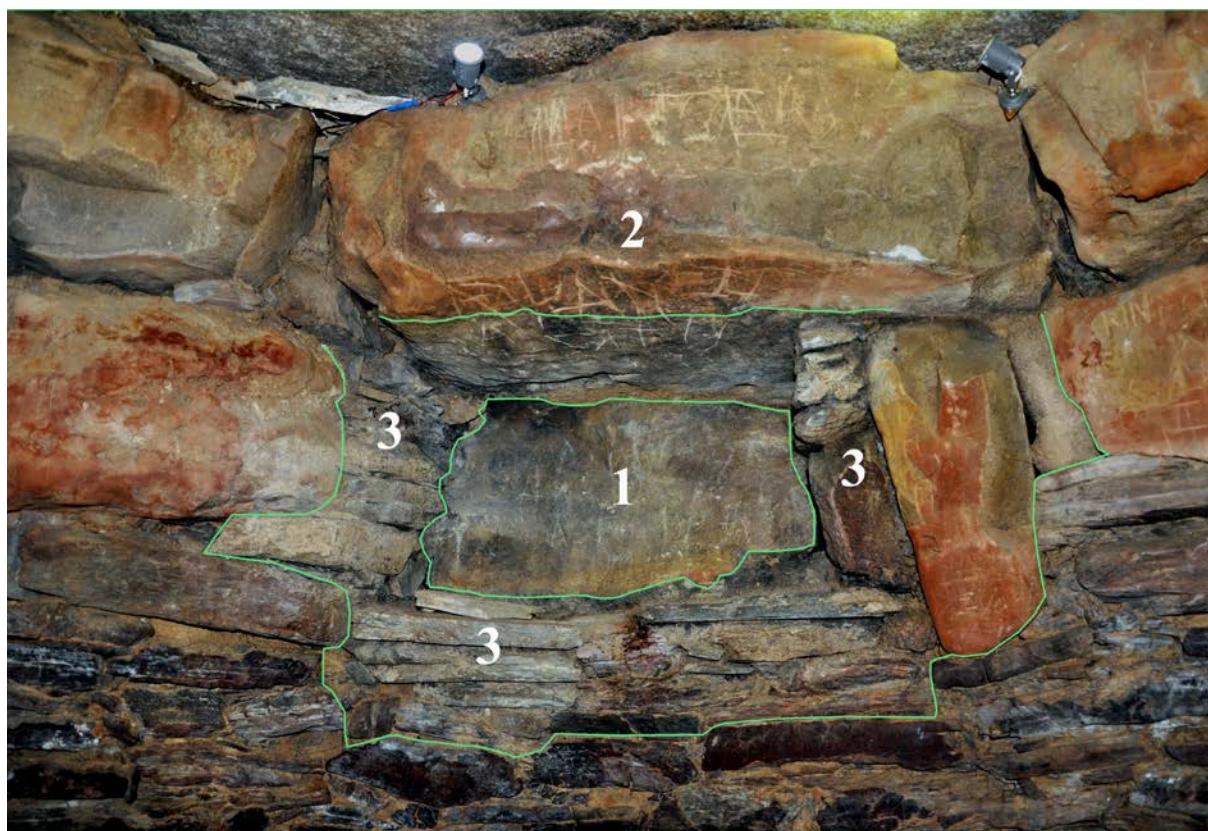
Figura 13. Hornacina de la cámara con indicación de elementos registrados durante el análisis constructivo.
