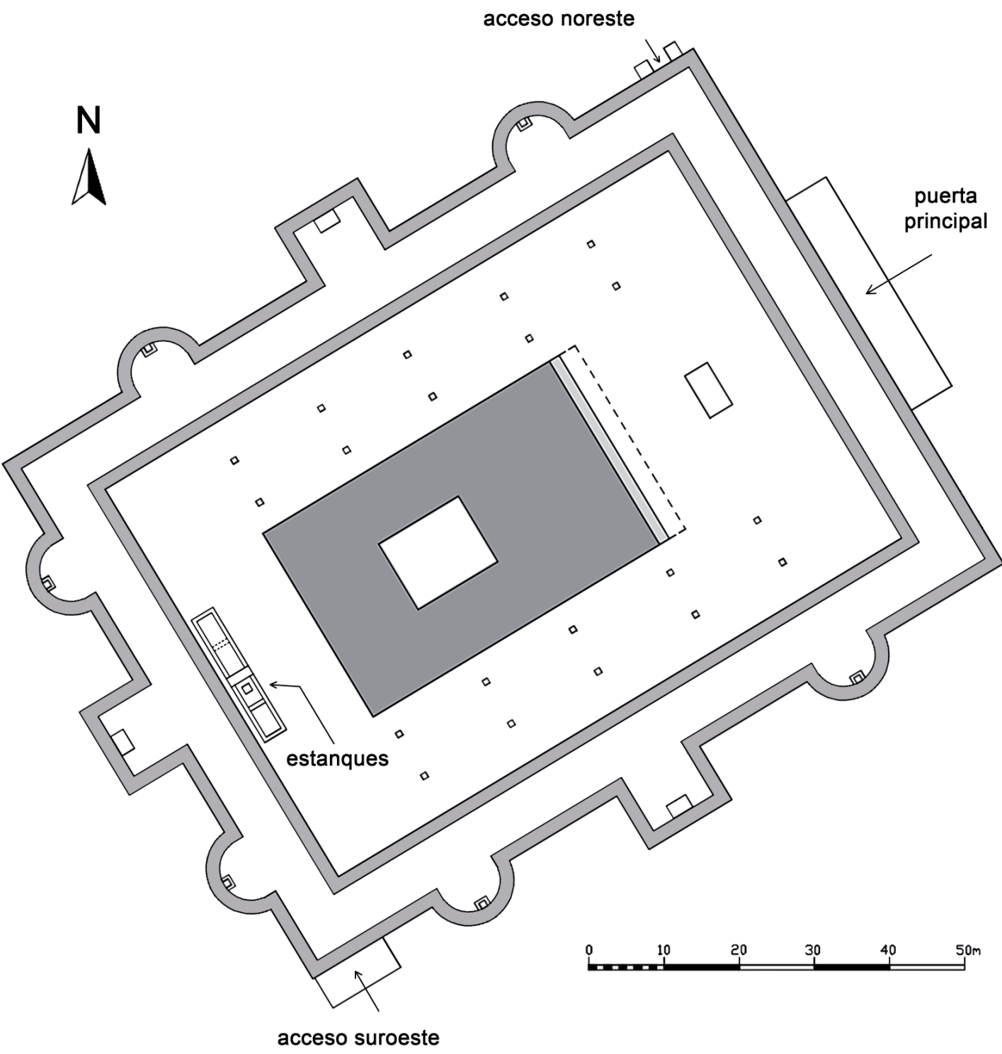
Figura 2. Planta del edificio conocido como Traianeum , en la ciudad romana de Italica , con el norte en el extremo distal de la imagen. Plano que incorpora medidas corregidas, elaborado por S. Vargas-Vázquez.
